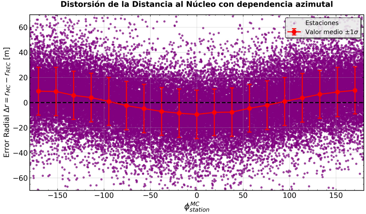
Figura 6.7: Distorsión de la coordenada radial de las estaciones del Infill en función del ángulo azimuthal. La modulación armónica demuestra que el núcleo reconstruido no sufre un esparcimiento aleatorio, sino un corrimiento sistemático a lo largo del eje temprano-tardío.
