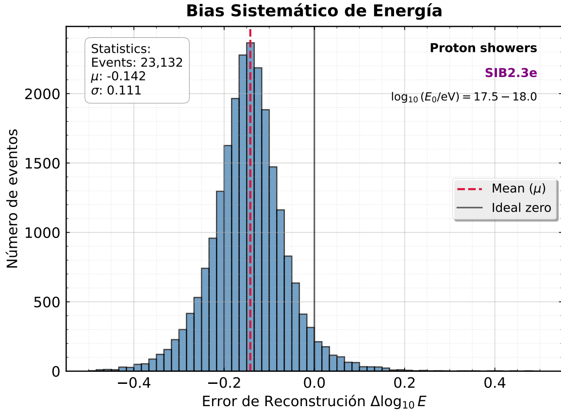
Figura 5.2: Histograma del error relativo en la reconstrucción de energía, \Delta \log_{10} E = \log_{10} E_{\text{REC}} - \log_{10} E_{\text{MC}} . La distribución presenta un valor central de \mu \approx -0,142 con una resolución de \sigma \approx 0,111 .
