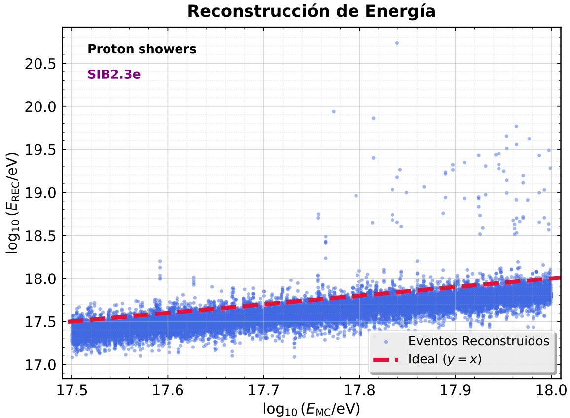
Figura 5.1: Reconstrucción de la energía del primario incidente. La línea punteada indica la relación ideal donde la energía reconstruida iguala a la simulada ( E_{\text{REC}} = E_{\text{MC}} ). Se observa la dispersión de los datos reconstruidos con una clara tendencia a subestimar el valor real.
