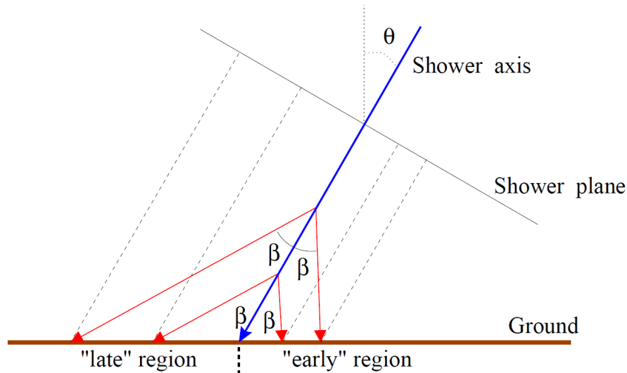
Figura 4.2: Esquema geométrico de cómo es la dispersión de las partículas con el ángulo de emisión respecto al eje de la lluvia \alpha (en la imagen llamado \beta ). Se ve que para un mismo ángulo de emisión, se alcanza una región mucho más tardía que temprana.
