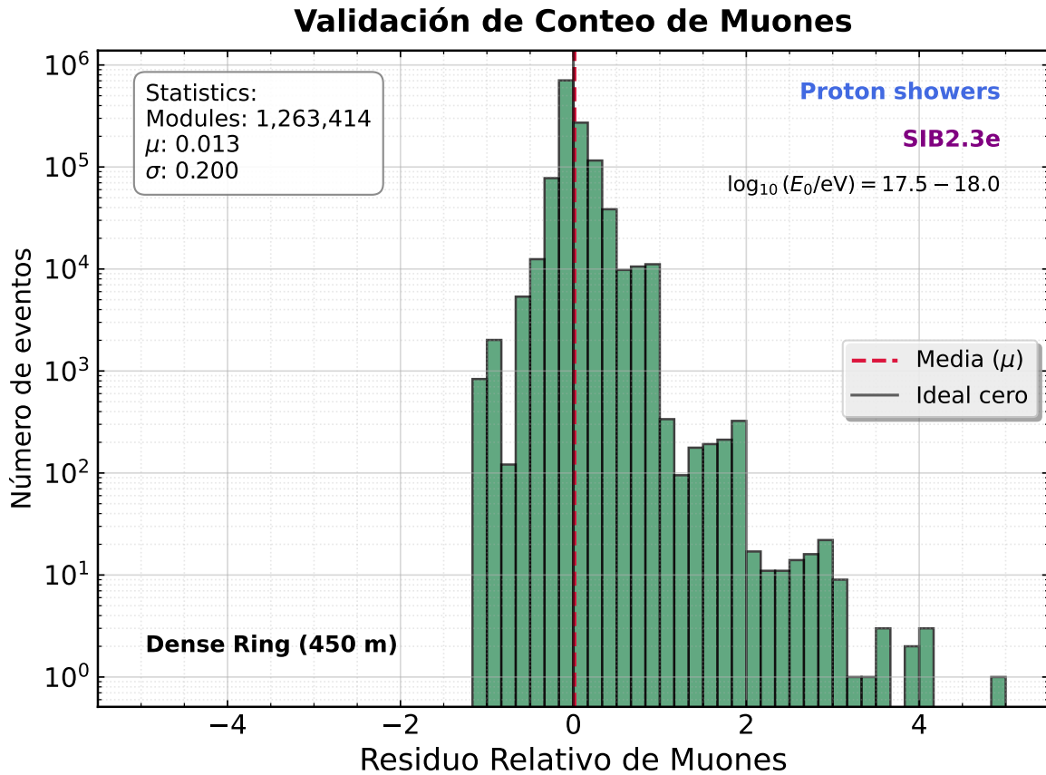
Figura 6.4: Distribución del residuo relativo en la reconstrucción de muones. Aunque la media es cercana a cero, se observa una asimetría intrínseca con una cola extendida hacia la sobre-reconstrucción de partículas.
