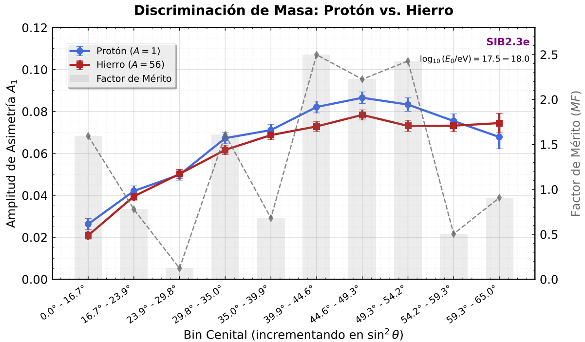
Figura 6.11: Evolución del Factor de Mérito ( MF ) en función del ángulo cenital. Se identifica un Sweet Spot de máxima separación entre bins de 40^\circ y 55^\circ , donde el poder de discriminación alcanza su máximo antes de degradarse por efectos instrumentales.
