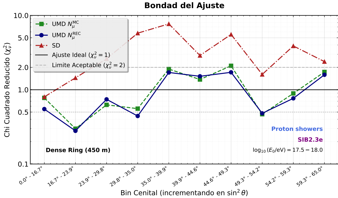
Figura 6.3: Bondad de ajuste \chi^2_\nu para los bins cenitales. Se observa que los ajustes del UMD (REC y MC) se mantienen cercanos a la unidad, mientras que el SD presenta valores elevados debido a la alta precisión estadística de la muestra.
