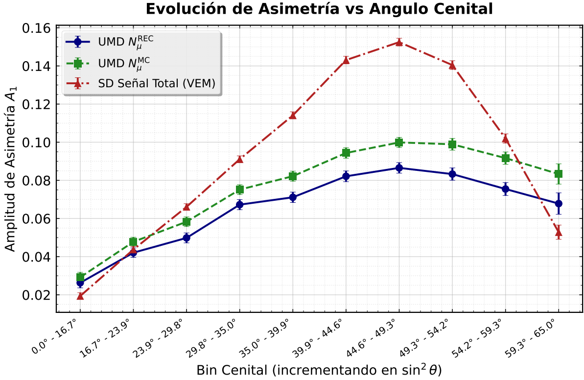
Figura 6.2: Evolución de la amplitud A_1 con su error en función de \theta para el UMD (REC en azul, MC en verde) y el SD (rojo). Se observa la inversión de dominancia entre el SD y el UMD a altas inclinaciones.
