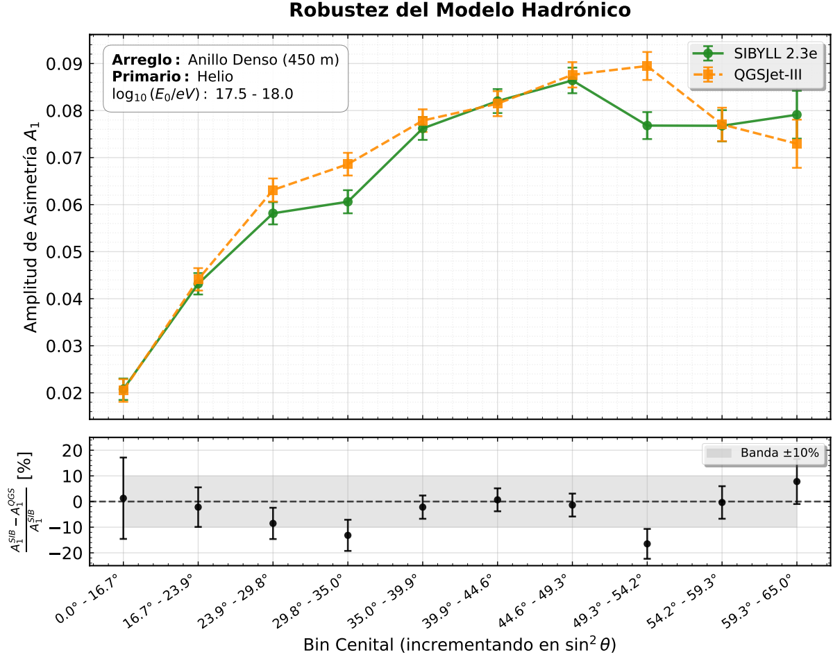
Figura 6.9: Comparación de la amplitud A_1 para lluvias de Helio simuladas con diferentes modelos hadrónicos. El panel inferior muestra que la diferencia relativa se mantiene mayoritariamente dentro de una banda de tolerancia aceptable, indicando una tendencia común independiente del modelo.
