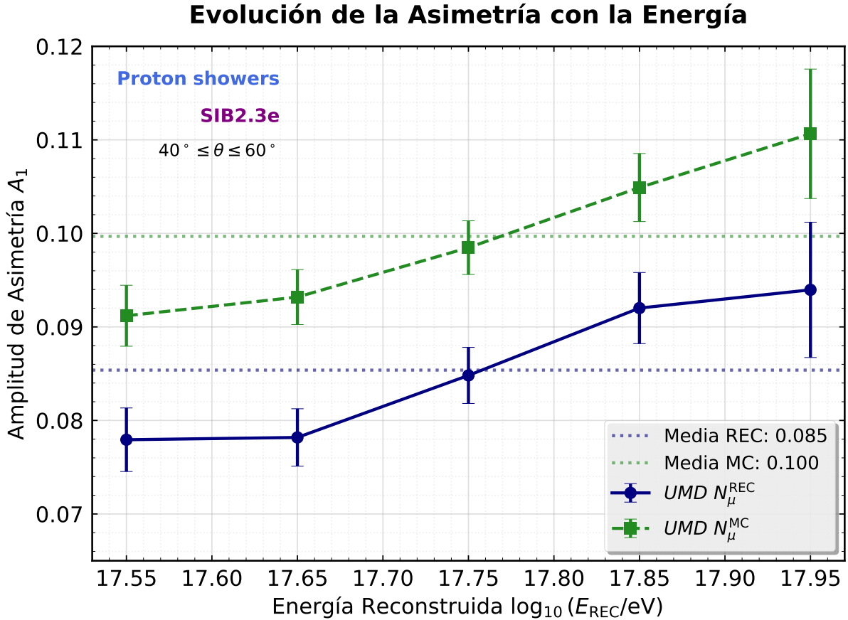
Figura 6.10: Evolución de la amplitud de asimetría A_1 en función de la energía reconstruida para cascadas de protón simuladas con SIBYLL 2.3e. Se observa un leve incremento lineal en la asimetría a mayores energías, presente tanto a nivel Monte Carlo como en la reconstrucción.
