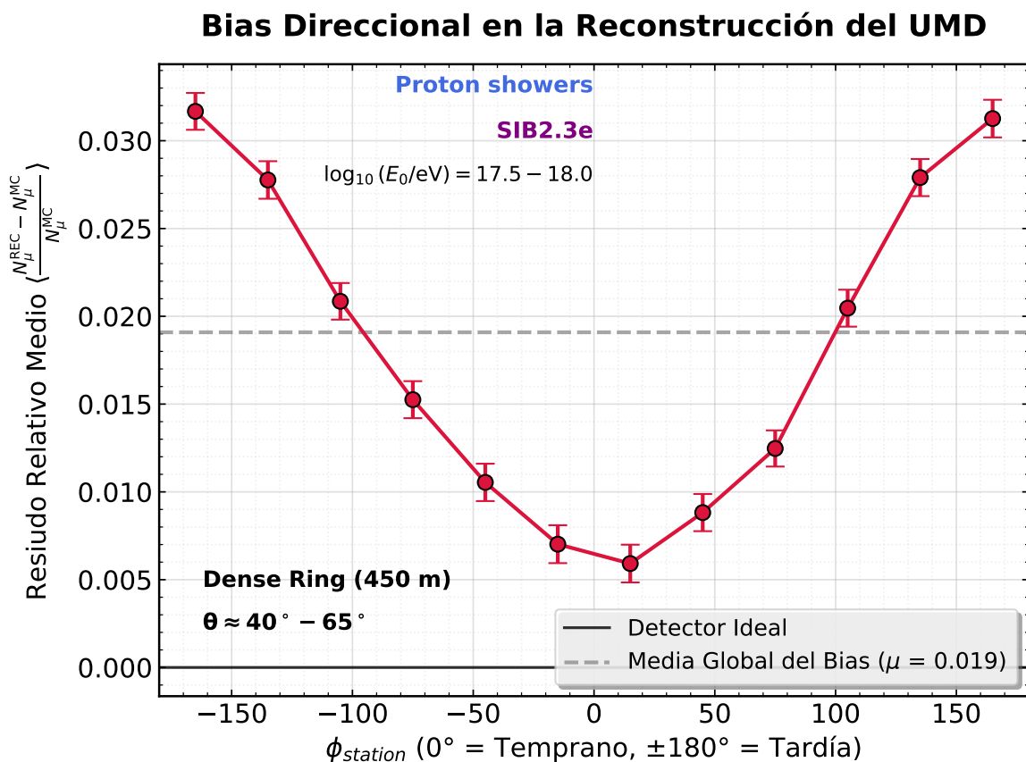
Figura 6.5: Distribución de la media del residuo relativo de reconstrucción en función del ángulo azimutal de la estación en el plano de la lluvia. Se evidencia un desempeño degradado en las regiones tardías ( \pm 180^\circ ), donde el sesgo de sobreconteo es máximamente superior al de la región temprana ( 0^\circ ).
